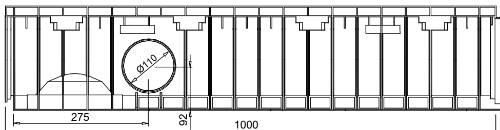
Поглед странично
