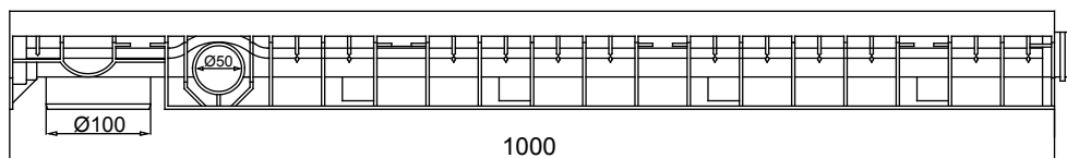
Поглед странично
