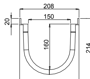
Сечение улей
