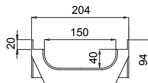
Сечение улей
